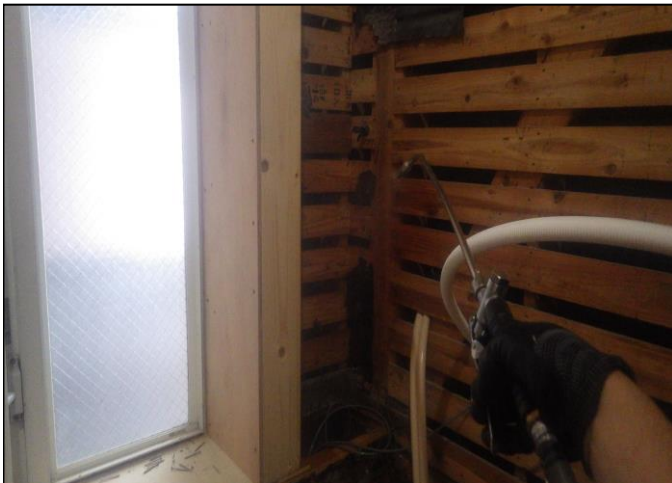
壁面: 木部処理剤吹付け
